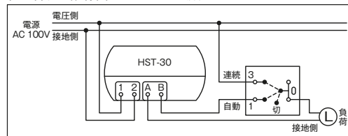
組み合わせ配線図 HST-30 PW の場合
