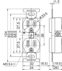
接地形埋込ダブルコンセント 15A-125V 1132
