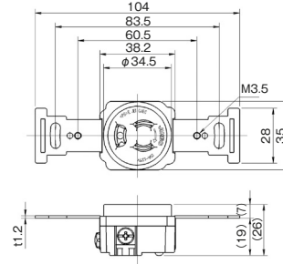
抜止接地形埋込コンセント 1138
