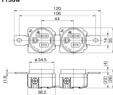
埋込接地形コンセント 125V 1136W
