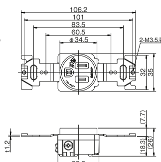
接地埋込コンセント 2極接地極付 15A-125V H1136
