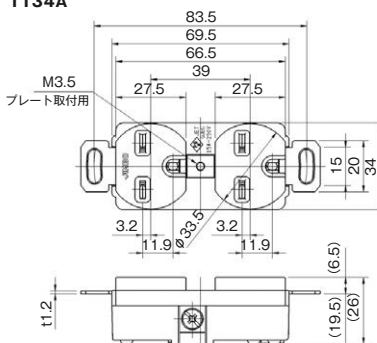
埋込接地形ダブルコンセント 250V
