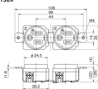
埋込接地形コンセント 125V 1136X
