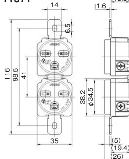
埋込接地形コンセント 250V 1137Y
