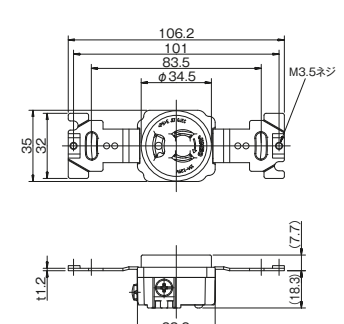
抜止接地埋込コンセント 2極接地極付 15A-125V H1138
