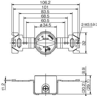
埋込コンセント 2極 15A-125V H1071
