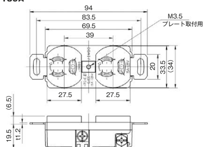
抜止接地形埋込ダブルコンセント
