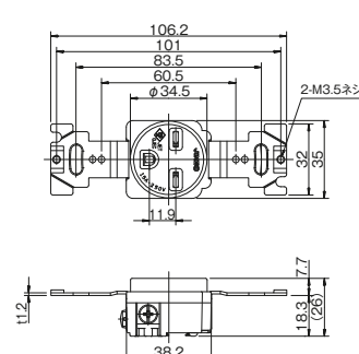
接地埋込コンセント 2極接地極付 15A-250V H1137
