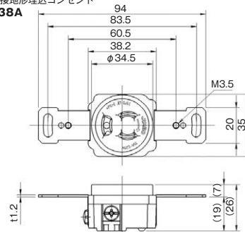
抜止接地形埋込コンセント
