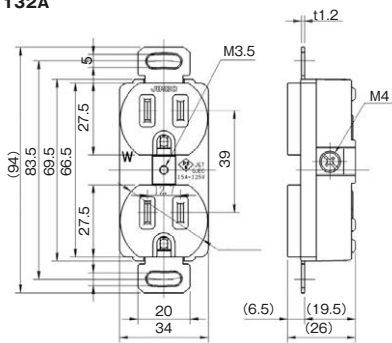
埋込接地形ダブルコンセント 125V
