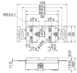
接地形埋込ダブルコンセント 15A-250V 1134
