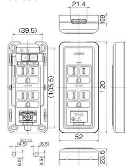
露出形アースターミナル付接地コンセント ダブル CS-55GE PW
