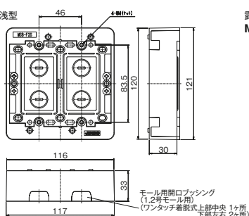
露出ボックス 2 連用 浅型 MSB-F2S
