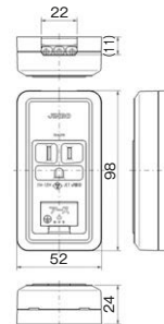
露出形アースターミナル付接地コンセント シングル CS-5GE PW
