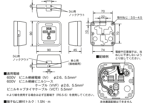
露出ボックス 1 連用 標準型 MSB-F1
