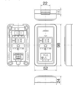
露出形アースターミナル付接地コンセント 15A・20A兼用 CS-ITGE PW
