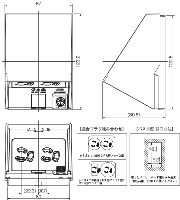
寸法図
