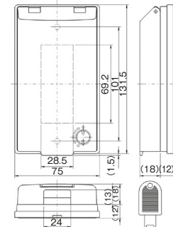
防滴プレート キー付き3個用 樹脂製 BPN-3UWKY
