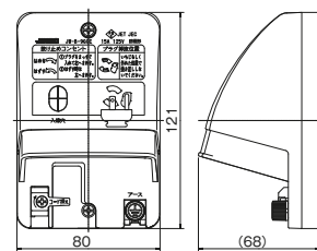
防雨形入線機能付抜止接地コンセント2極接地極付 JW-B-9GCE
