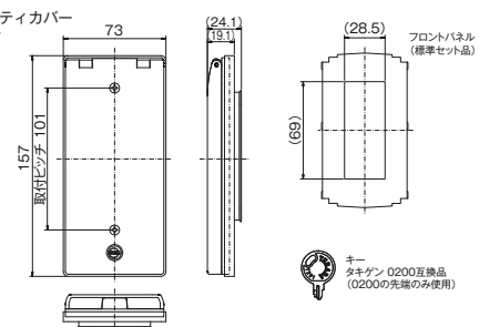
防滴プレート キー付き3個用 樹脂製 BPN-3UWKY
