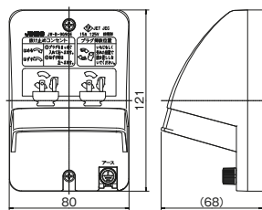
防雨形抜止接地ダブルコンセント2極接地極付 JW-B-9G9GE
