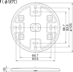
エレガンス丸形 blanks プレート 丸形 BPN-0UR PW BPN-TUR PW (φ9穴)
