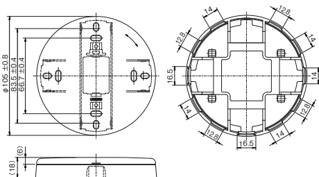
エレガンス丸形 blanks プレート 丸形 BPN-0UR PW BPN-TUR PW (φ9穴)
