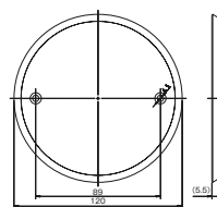
丸形blankプレート 大丸形 843S
