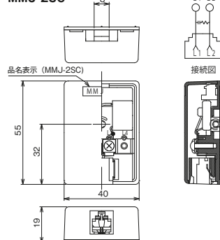
露出形モジュラジャック コンデンサ付 6極2心用 MMJ-2SC
