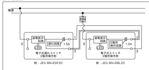
標準結線図
