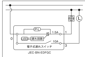
標準結線図
