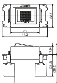
チェック用 オーロラマークスイッチ本体 3路 2線式 JEC-BN-3MLCR PW
