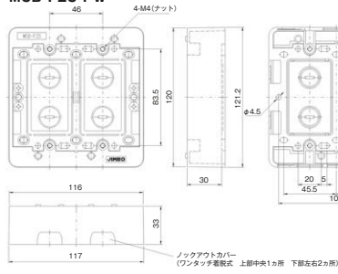
露出ボックス 2 連用 浅型 MSB-F2S PW
