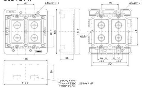
露出ボックス 2 連用 標準型 MSB-F2 PW
