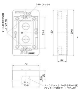
露出ボックス 1 連用 極浅型 MSB-F1SS PW
