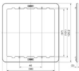
継棒 2 連用 高さ3mm BAN-3-2 PW
