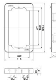
継棒 1 連用 高さ13mm BAN-13-1 PW
