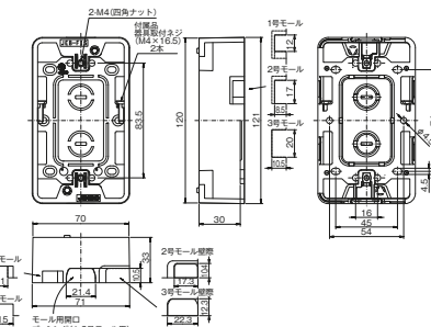
露出ボックス 1 連用 浅型 JEB-F1S PW
