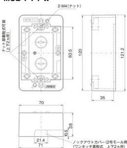
露出ボックス 1 連用 標準型 MSB-F1 PW
