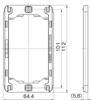
取付台座 1 連用 WJB-1
