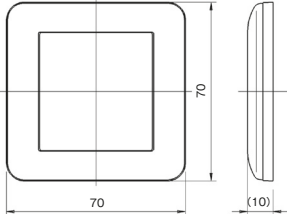
取付台座 3 連用 WJB-3
