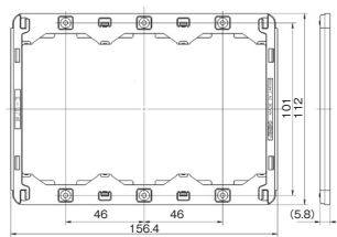
取付台座 3 連用 WJB-3
