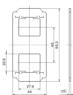
気密パッキン 2口用 WJX-C2
