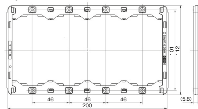
取付台座 5 連用 WJB-5
