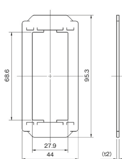
気密パッキン 3口用 WJX-C3
