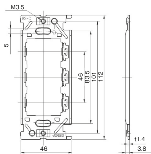
埋込取付枠 金属枠 BS-C
