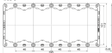
取付台座 5 連用 WJB-5
