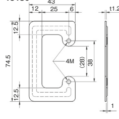
取付台座 4 連用 WJB-4
