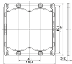
取付台座 2 連用 WJB-2
