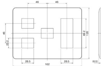
コンセントプレート 5 連用 WJE-00000
