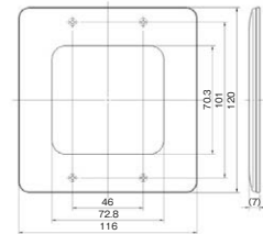
2 ピースコンセントプレート 3 連用 WJD-000
