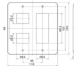
2 ピースコンセントプレート 2 連用 WJD-23
