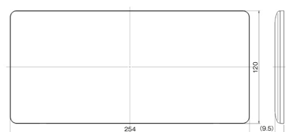
コンセントプレート 5 連用 WJE-00000
