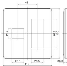
コンセントプレート 4 連用 WJE-0000
