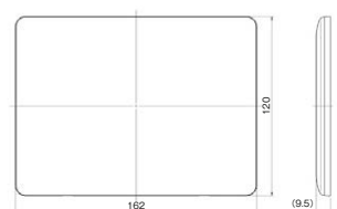
コンセントプレート 3 連用 WJE-000
