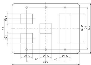
blankプレート 取付枠付 1 連用 WJ90001PW
