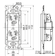
ねじ締め式
