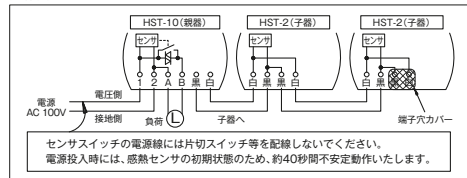
配線図
