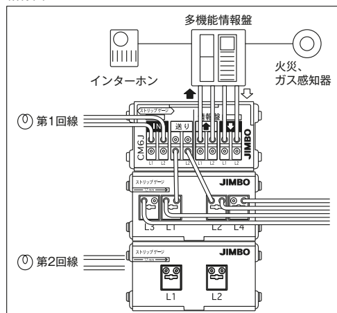
結線図
