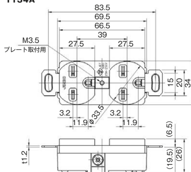
埋込接地形ダブルコンセント 250V
