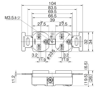
接地形埋込ダブルコンセント 15A-250V 1134
