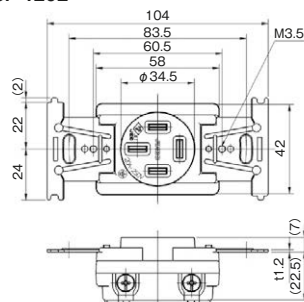
接地埋込コンセント 3P E (旧4P) 20A CF-4202
