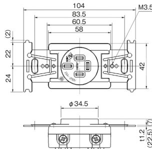
接地埋込コンセント 3P E (旧4P) 15A CF-4152
