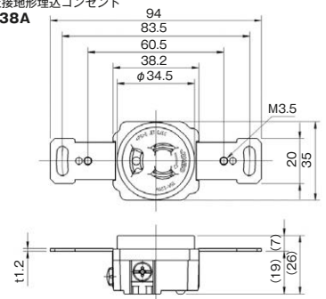
抜止接地形埋込コンセント
