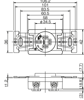
接地埋込コンセント 2極接地極付 15A-250V H1137
