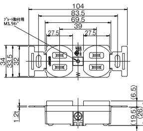
埋込式コンセント 2極 15A-125V 1060
