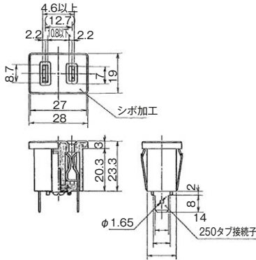
機器用 はめ込コンセント 1341
