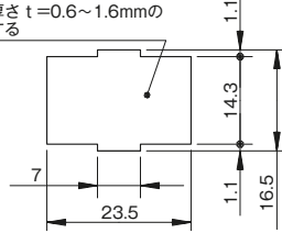
パネル穴あけ寸法
