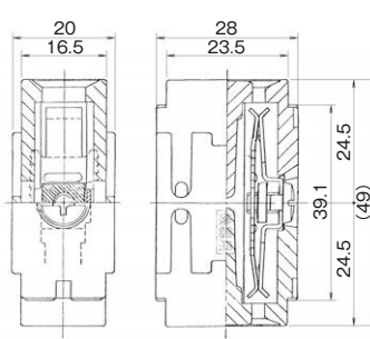
両口コンセント 1288
