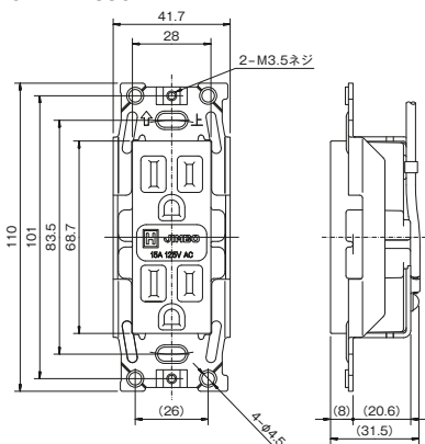
医用 埋込接地ダブルコンセント JME-BN-55GH
