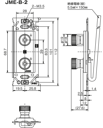
医用 接地端子 JME-B-2
