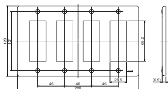
4連用 BP-3A-4
