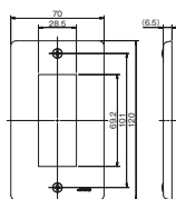
1 連用 BP-3A
