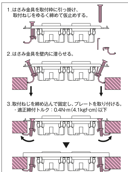
はさみ金具を使用した施工
