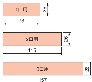
はさみ金具を使用した施工の開口寸法
