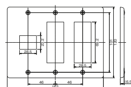
3連用 BP-1+3A-2
