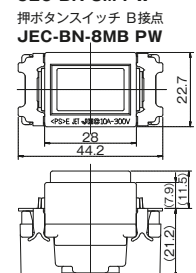
押ボタンスイッチ A接点 JEC-BN-8M PW 押ボタンスイッチ B接点 JEC-BN-8MB PW
