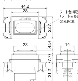
パイロットランプ 電流検知形 0.5A用 JEC-BN-6CL PW
