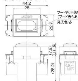
パイロットランプ 電流検知形 4A用 JEC-BN-6CR PW
