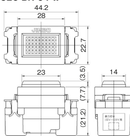
パイロットランプ 電圧検知形 JEC-BN-6 PW
