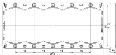
取付台座 5連用 WJB-5
