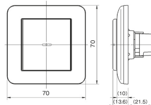
ミニプレート組み合わせ例 SWJ101PW
