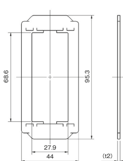
気密パッキン 3口用 WJX-C3
