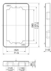
縦枠1連用 高さ13mm BAN-13-1 PW
