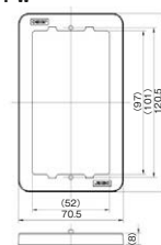
縦枠1連用 高さ8mm BAN-8-1 PW
