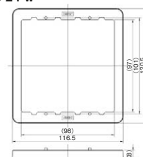
縦枠2連用 高さ8mm BAN-8-2 PW
