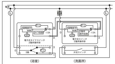
換気扇2箇所操作結線例
