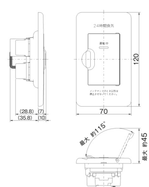
24時間換気用メインスイッチ エレガンスタイプ 換気扇スイッチ+風量切換スイッチ VBN-23L PW
