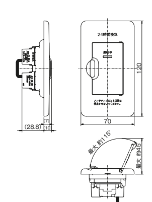
24時間換気用メインスイッチ エレガンスタイプ 換気扇スイッチ+風量切換スイッチ VBN-13L PW VBN-33L PW
