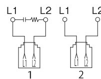
接続図
