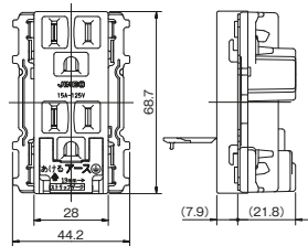
アースターミナル付 接地ダブル JEC-BN-55GEK PW
