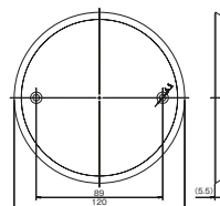
丸形フランクプレート 大丸形 843A
