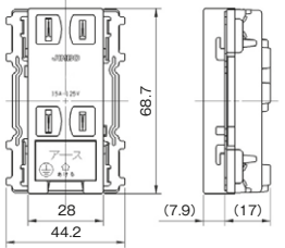
ダブル (2コモジュール) EG-55 PW
