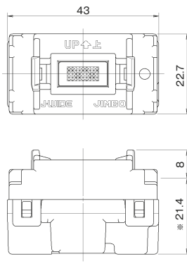
パイロットランプ 電流検知形 0.5A用 WJ-6CL
