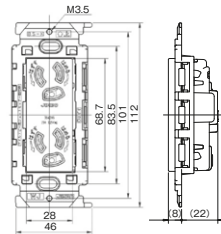
抜止接地ダブル 絶縁枠 JEC-BN-99GV PW
