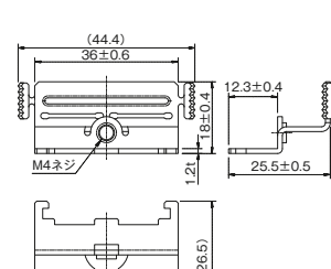
はさみ金具 上下形 18~21mm用 WJS-H18
