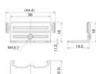
はさみ金具 上下形 9~15mm用 WJS-H12
