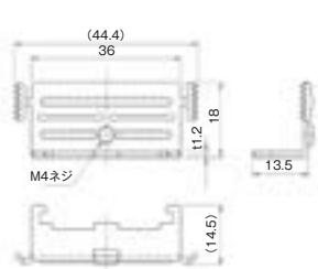
はさみ金具 上下形 3~9mm用 WJS-H6
