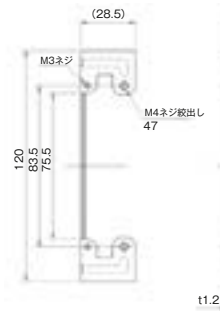
はさみ金具 ボード用C形 8500M
