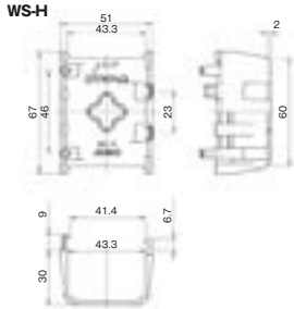
J-WIDE専用 保護カバー WS-H
