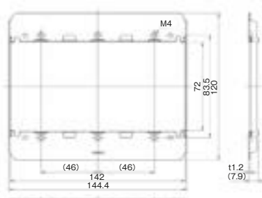
はさみ金具 保護カバーワンタッチ取付用 3連用 8653CT
