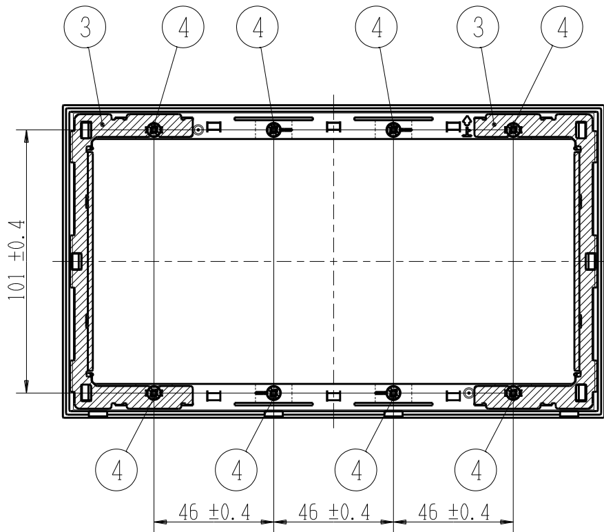
カバープレート未装着図 (1/2)
