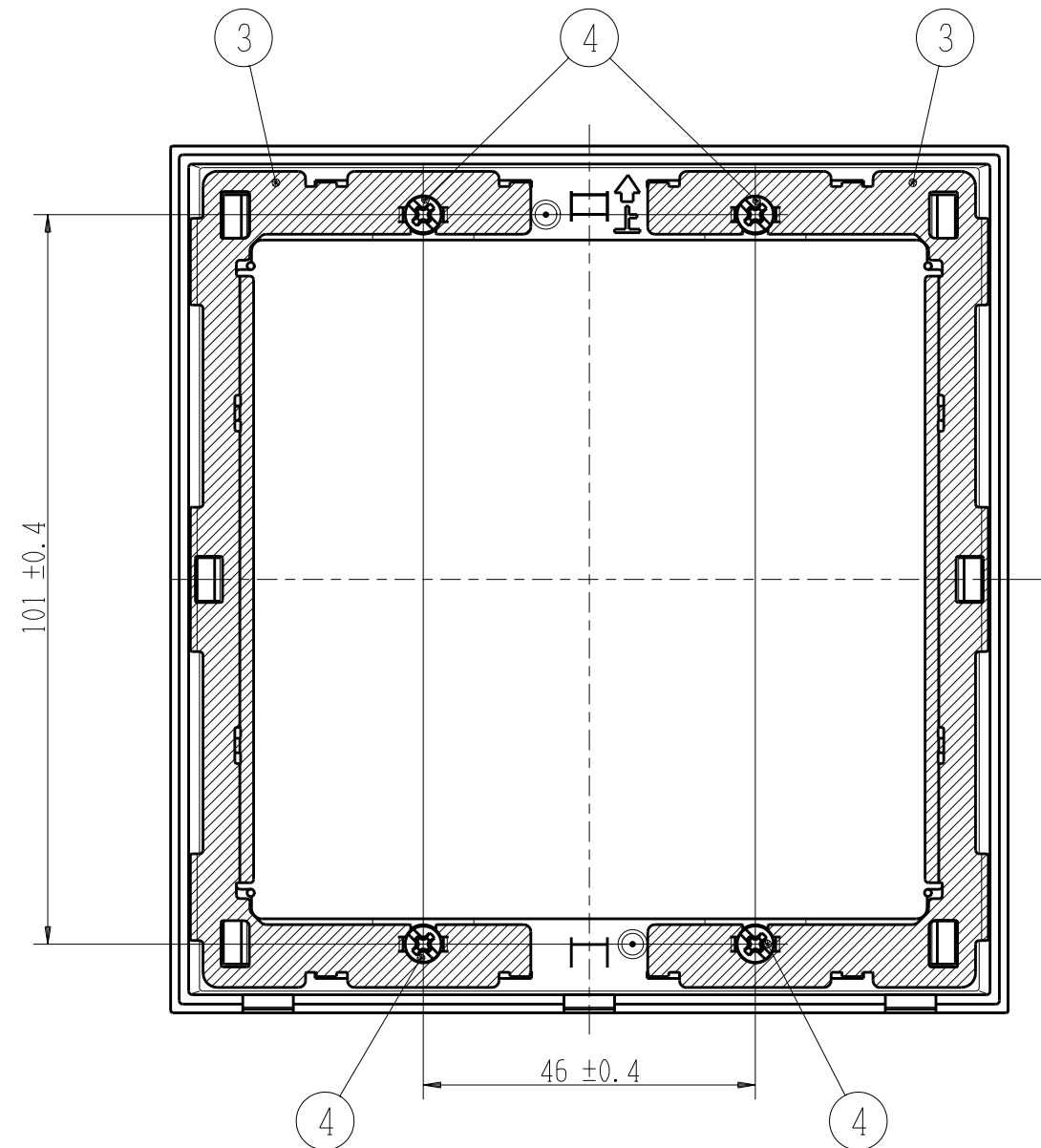
カバープレート未装着図
