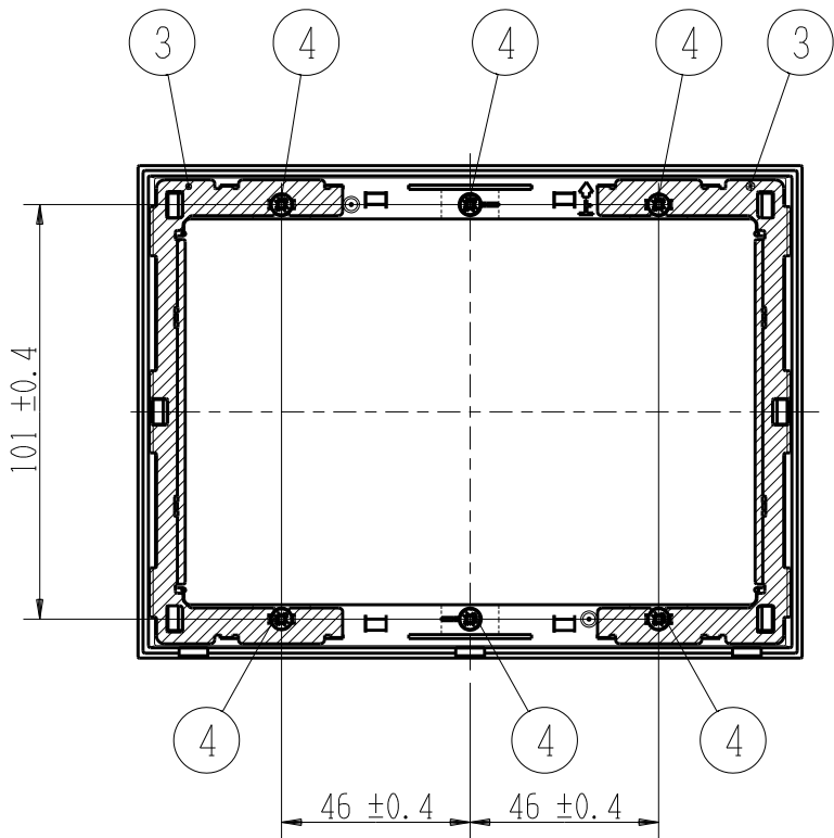
カバープレート未装着図 (1/2)
