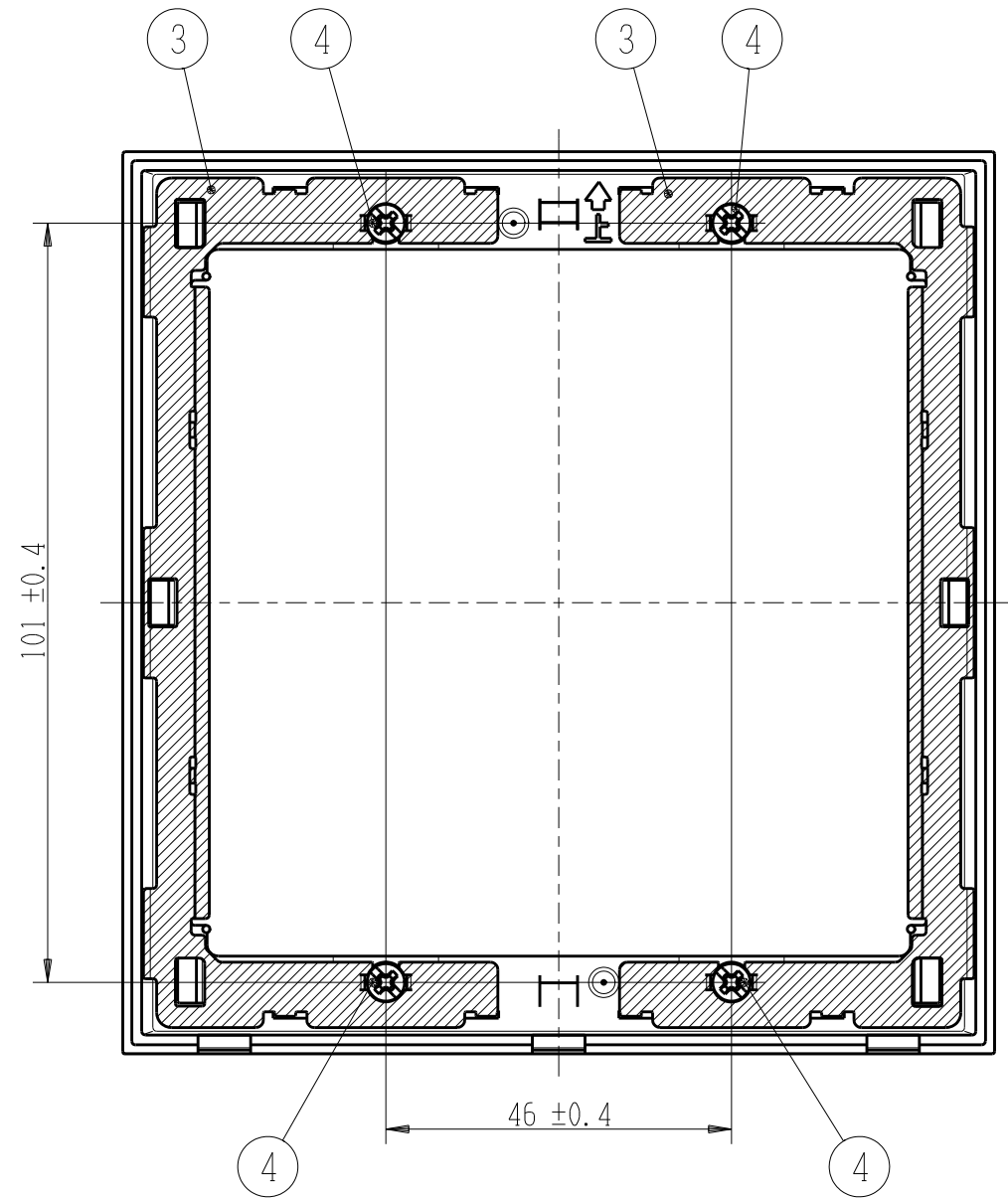
カバープレート未装着図
