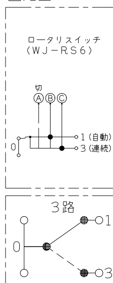
回路図
