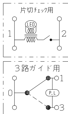
回路図
