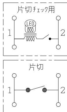
回路図
