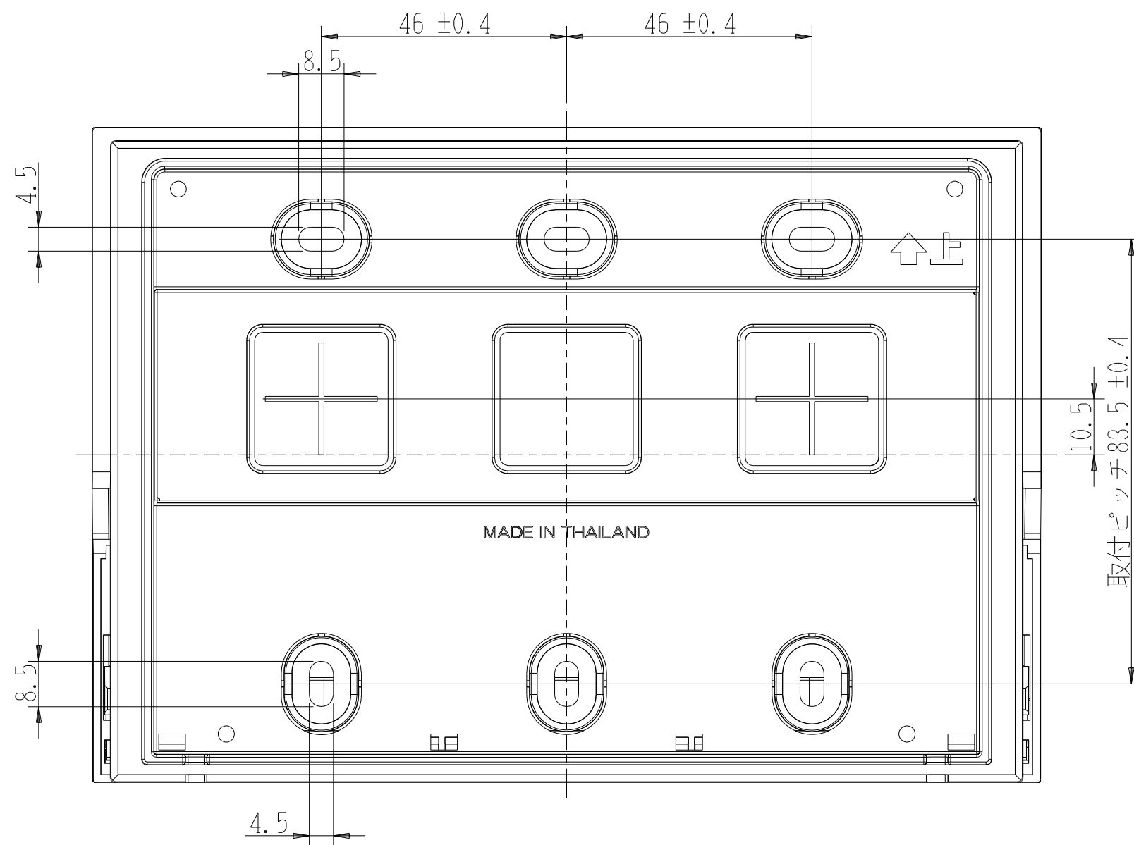
裏面図
