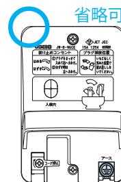
JW-B-9GCE (防雨形屋外コンセント)
