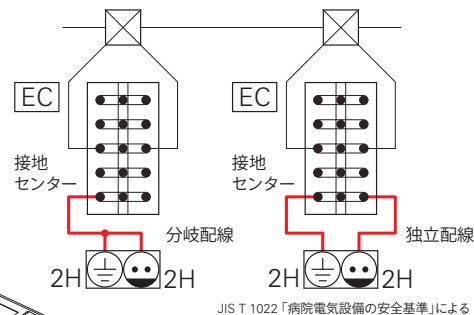
配線接続図（赤色太線部分を点検します）
