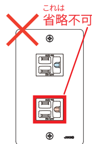
JW-B-9GCE (防雨形屋外コンセント)
